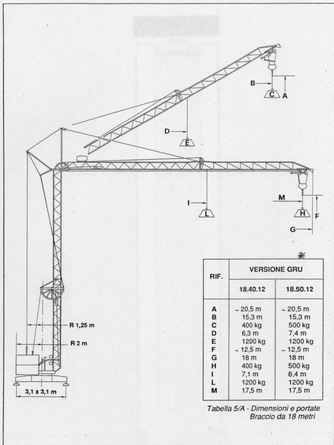
Fig. 1 (Foglio 1 di 3) - Braccio da 18 metri
