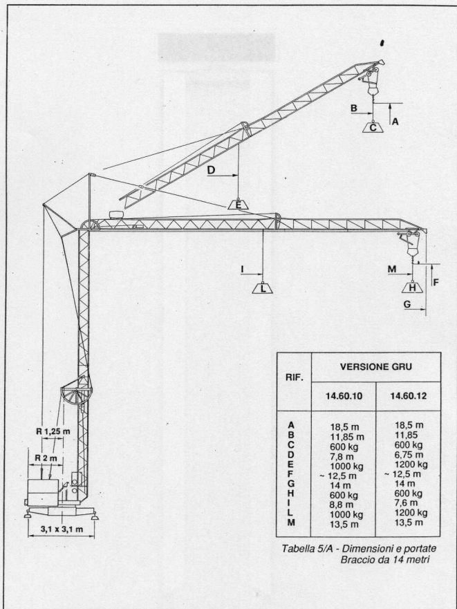
Fig. 1 (Foglio 1 di 2) - Braccio da 14 metri
